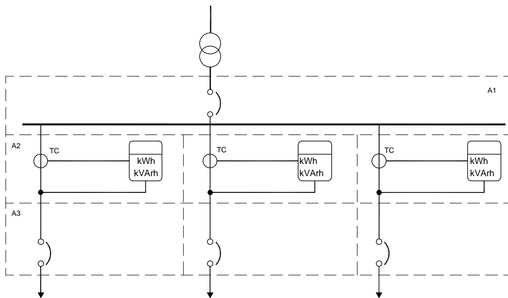
ARMARIO PARA MEDICIÓN SEMIDIRECTA VARIOS SERVICIOS
