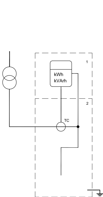
ARMARIO PARA MEDICIÓN SEMIDIRECTA
