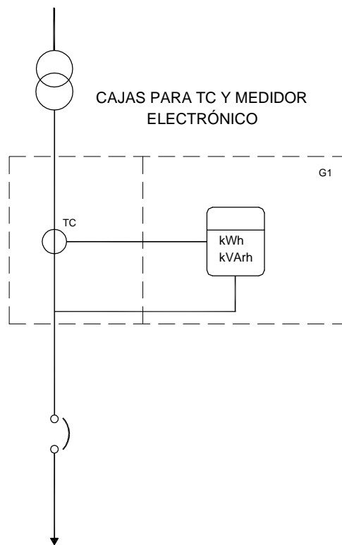
CAJAS PARA MEDICIÓN SEMIDIRECTA
