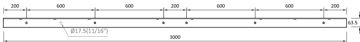
VISTA EN ALZADO Escala 1:20
